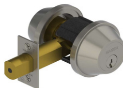
mod. 3214 Cerrojo llave/llave 2-3/4" Grado 2. US32D
